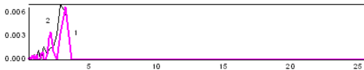
Hiệp phổ áp suất P với V_x (1) và V_y (2)
