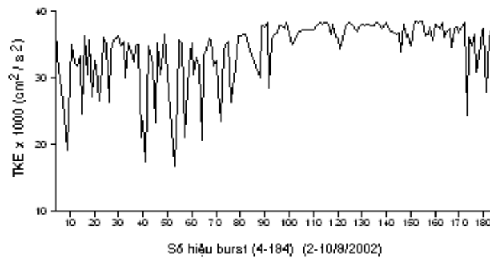
Biến thiên của động năng rối toàn phần theo các Burst quan trắc
