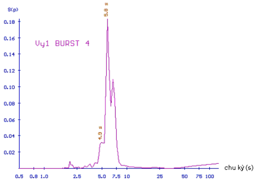
Phổ thành phần hướng bắc của dòng chảy, đầu đo 1
