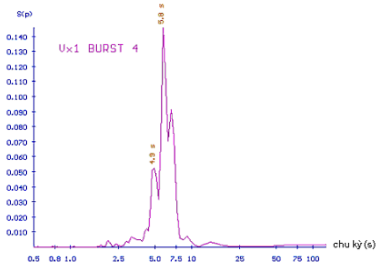
Phổ thành phần hướng đông của dòng chảy, đầu đo 1
