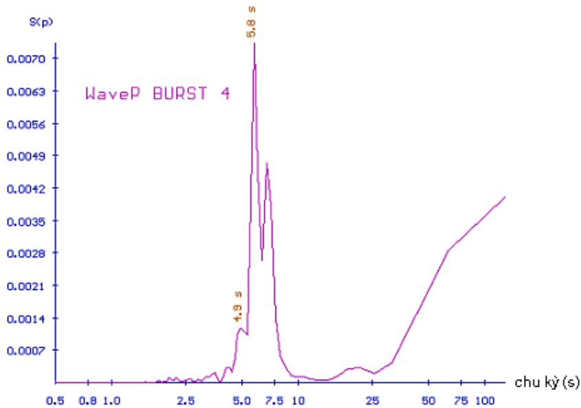
Phổ tần số áp suất sóng
