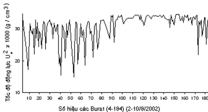
Biến thiên của tốc độ ma sát u * 2 theo các Burst quan trắc
