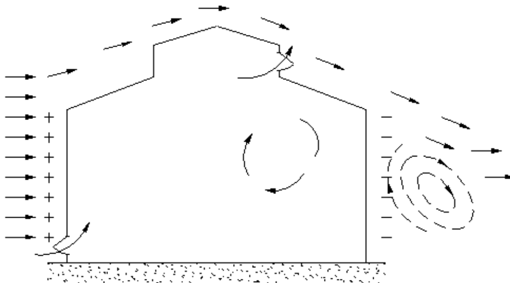
Phân bố áp suất dưới tác dụng của gió
