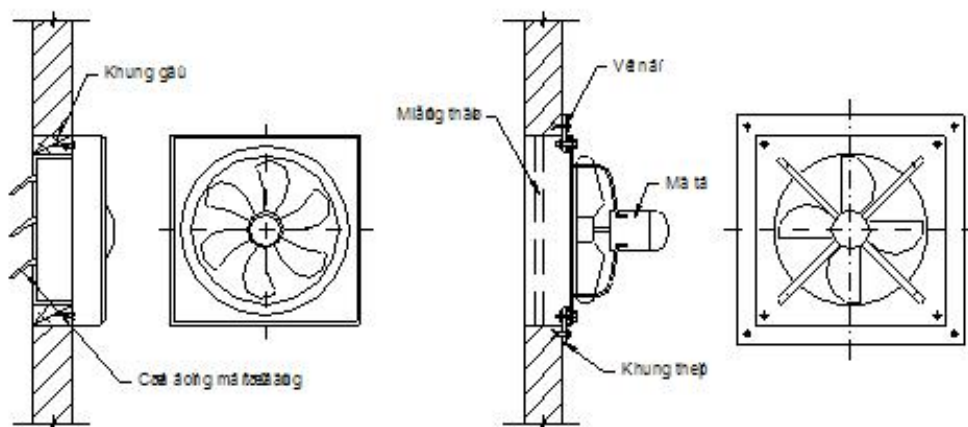
Lắp đặt quạt gắn tường
