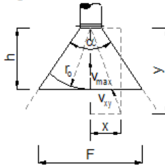
Luồng không khí trước chụp cường bức
