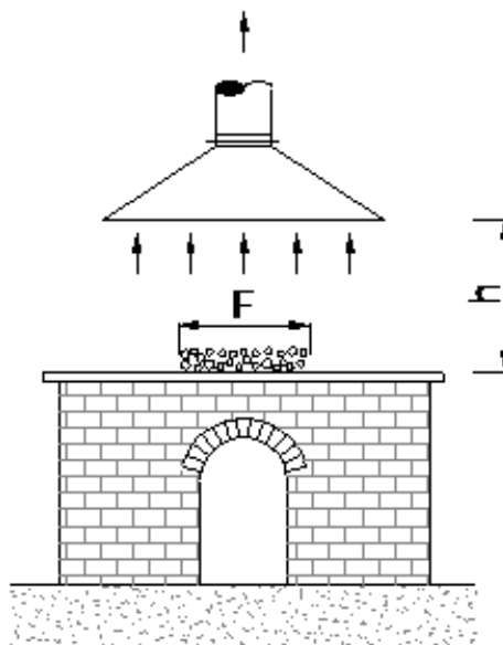
Chụp hút làm việc bằng sức hút tự nhiên
