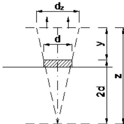
Luồng không khí bốc lên từ bề mặt toả nhiệt
