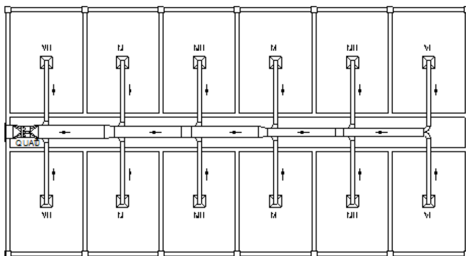
Sơ đồ bố trí quạt thông gió
