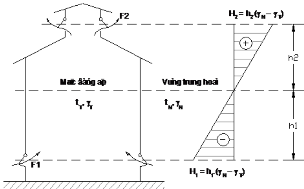
Nguyên lý thông gió do nhiệt áp
