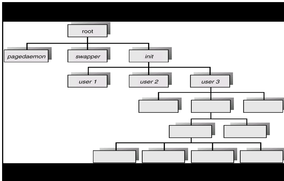
Hình III-7-Cây quá trình trên một hệ thống UNIX điển hình
