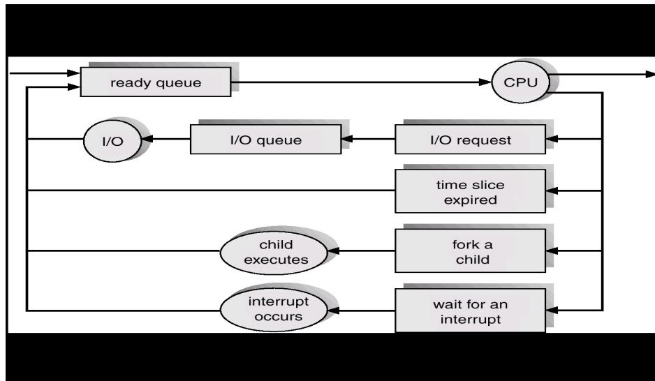
Hình III-5-Biểu diễn lưu đồ hàng đợi của lập thời biểu quá trình
