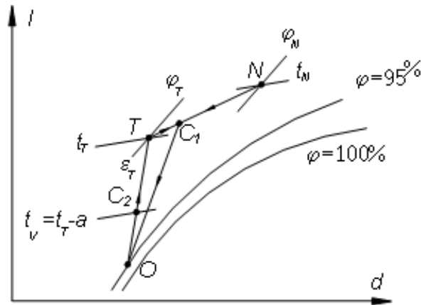
Biểu diễn sơ đồ tuần hoàn 2 cấp có điều chỉnh nhiệt độ trên I-d
