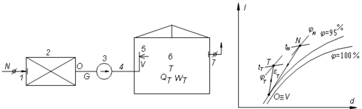
Sơ đồ nguyên lý và biểu diễn sự thay đổi trạng thái không khí trên đồ thị I-d
