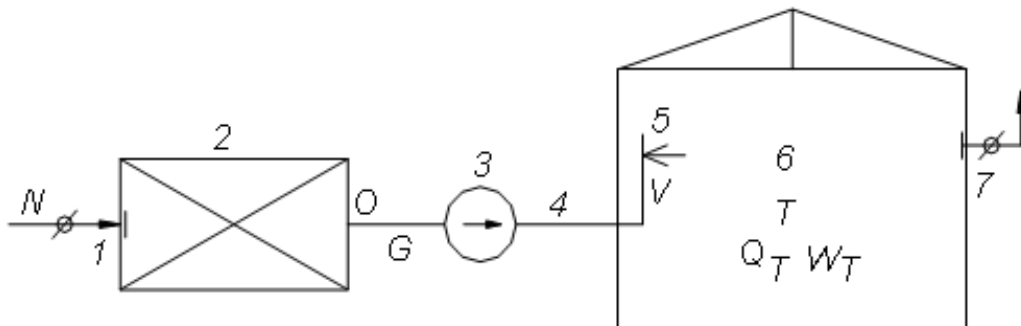
Sơ đồ thẳng mùa đông
