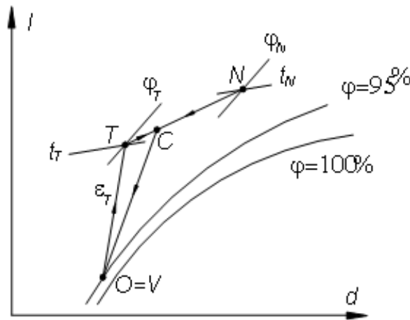
Biểu diễn sơ đồ tuần hoàn 1 cấp trên đồ thị I-d
