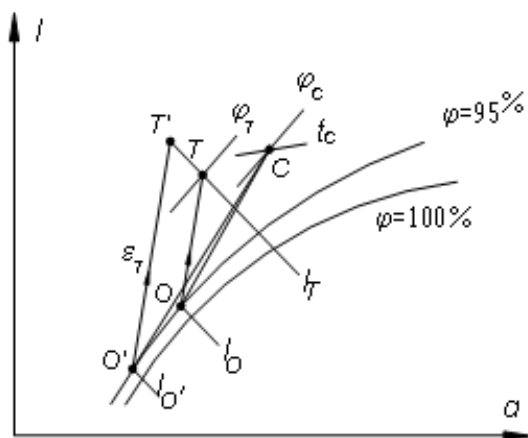
So sánh chu trình có và không có phun ẩm bổ sung
