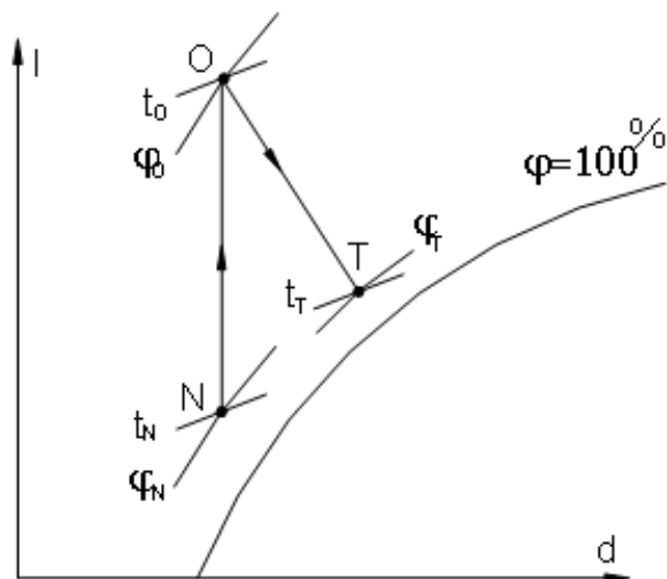
Biểu diễn sơ đồ tuần hoàn 1 cấp mùa đông trên đồ thị I-d
