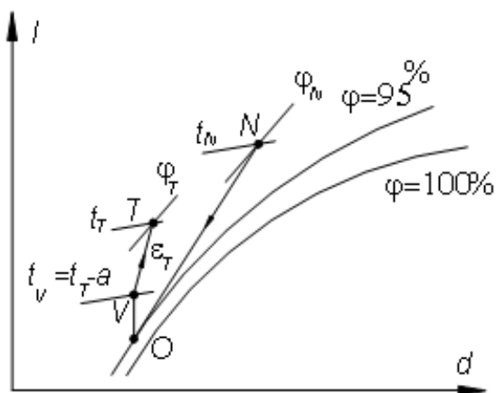
Sơ đồ thẳng khi nhiệt độ t v thấp
