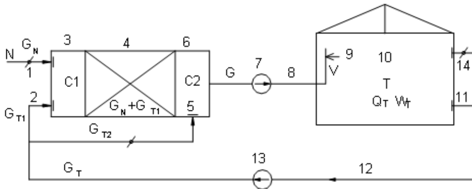
Sơ đồ tuần hoàn 2 cấp có điều chỉnh nhiệt độ
