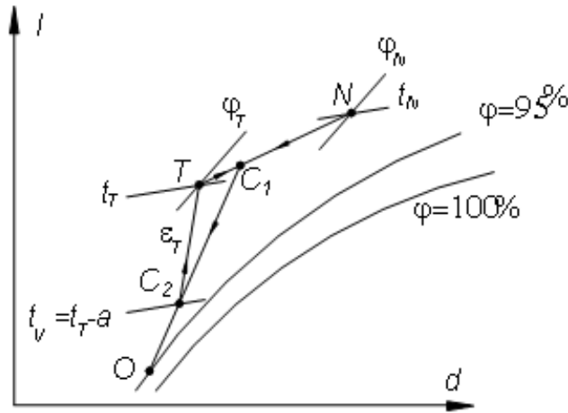
Sơ đồ tuần hoàn 2 cấp có điều chỉnh độ ẩm trên I-d
