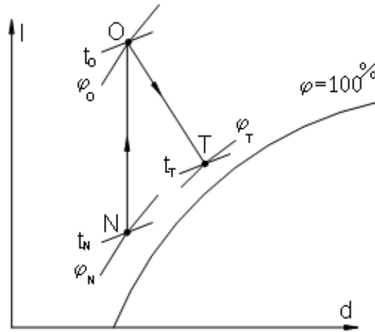
Biểu diễn sơ đồ thẳng mùa đông trên đồ thị I-d
