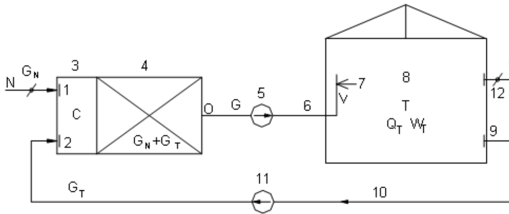
Sơ đồ tuần hoàn 1 cấp mùa đông
