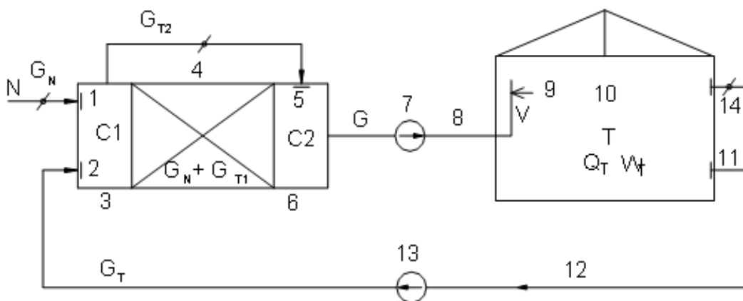
Sơ đồ tuần hoàn 2 cấp điều chỉnh độ ẩm
