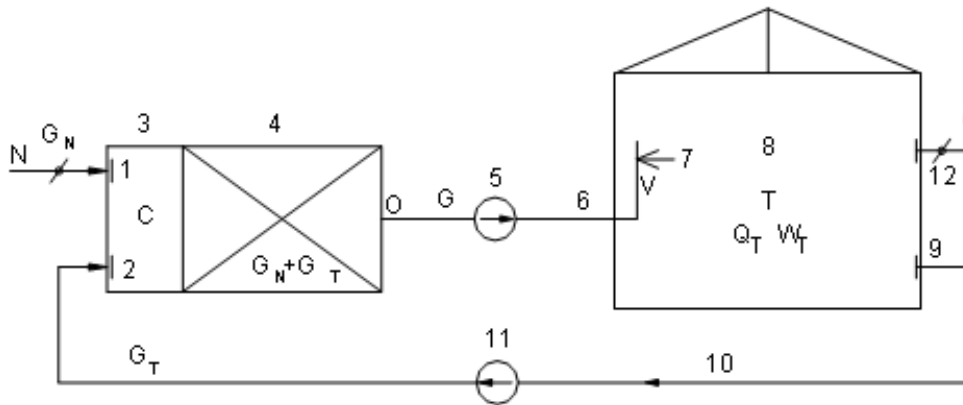
Sơ đồ tuần hoàn 1 cấp
