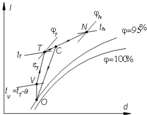
Sơ đồ tuần hoàn 1 cấp khi nhiệt độ t_V thấp
